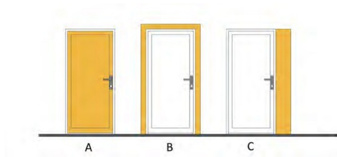
Ilustracja 60. Przykłady wyróżnienia drzwi na tle ściany: A – odmienne barwy drzwi i ściany, B – odmienne barwy ościeżnicy i ściany, C – dodanie akcentu kolorystycznego w formie pionowego pasa przy drzwiach od strony klamki, rys. Agnieszka Sowińska (opracowanie własne na podstawie „Modelu Dostępnej Szkoły”).
