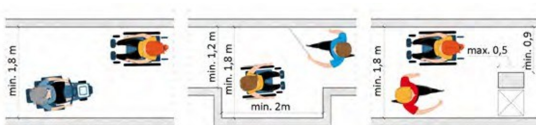
Ilustracja 53. Szerokości ciągów komunikacyjnych, rys. Katarzyna Guratowska i Maria Görlich-Opyd (opracowanie własne na podstawie „Modelu Dostępnej Szkoły”)
