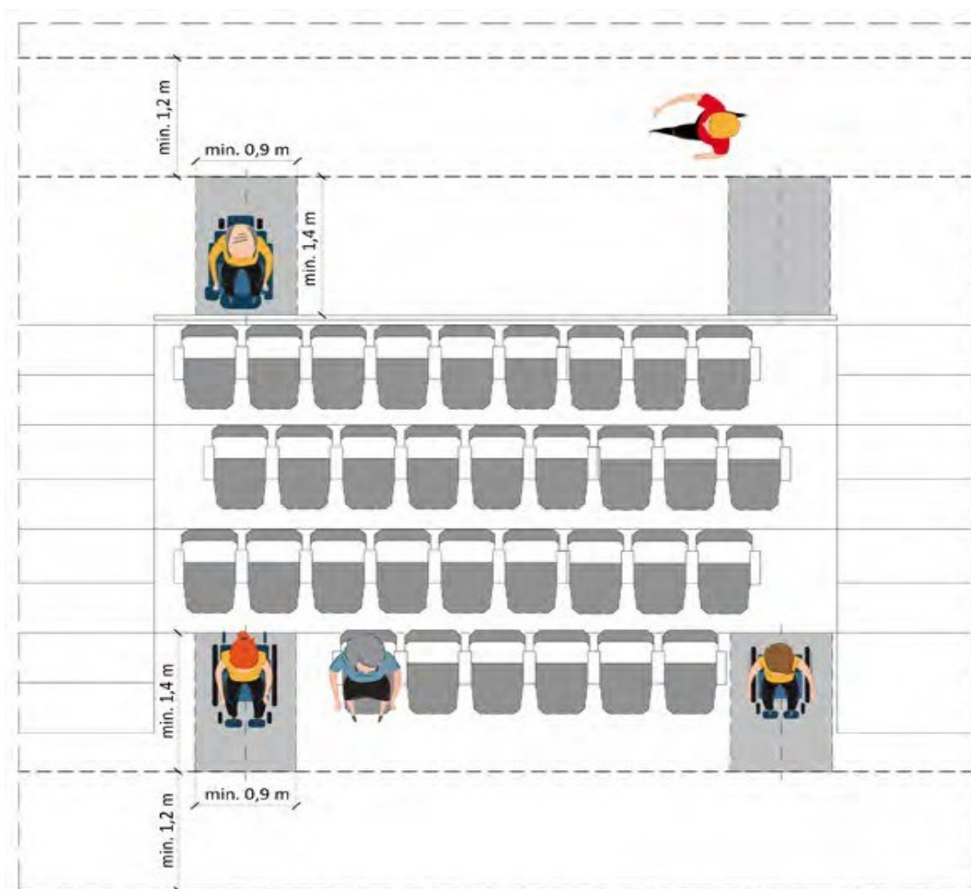
Ilustracja 93. Aranżacja miejsc dla osób na wózkach w obrębie widowni – rzut, rys. Agnieszka Sowińska i Maria Görlich-Opyd
