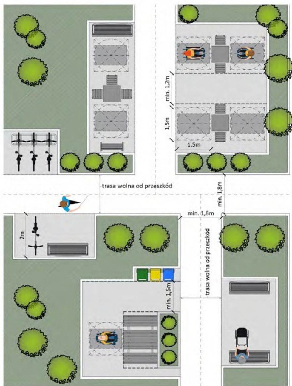
Ilustracja 30. Przykłady aranżacji miejsc wypoczynku na terenach rekreacyjnych, rys. Agnieszka Sowińska i Maria Görlich-Opyd
