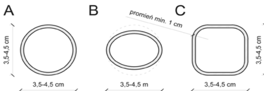
Ilustracja 43. Przykłady prawidłowych przekrojów poręczy, A – poręcz okrągła, B – poręcz owalna i C – poręcz prostokątna o zaokrąglonych narożnikach, rys. Katarzyna Guratowska (opracowanie własne na podstawie „Modelu Dostępnej Szkoły”)
