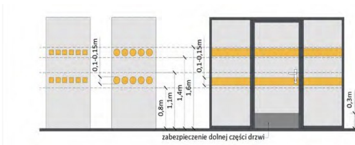
Ilustracja 51. Sposoby oznakowania elementów transparentnych takich jak ściany i drzwi, rys. Agnieszka Sowińska (opracowanie własne na podstawie „Modelu Dostępnej Szkoły”)
