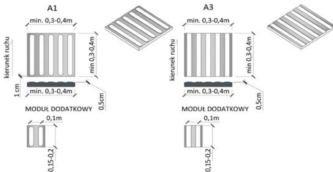
Ilustracja 6. Płytki kierunkowe do zastosowań: A1 – na zewnątrz i wewnątrz obiektów, A3 – do wnętrza i zadaszonych peronów zewnętrznych, rys. Agnieszka Sowińska (opracowanie własne na podstawie „Standardów dostępności dla polityki spójności 2021-2027”)
