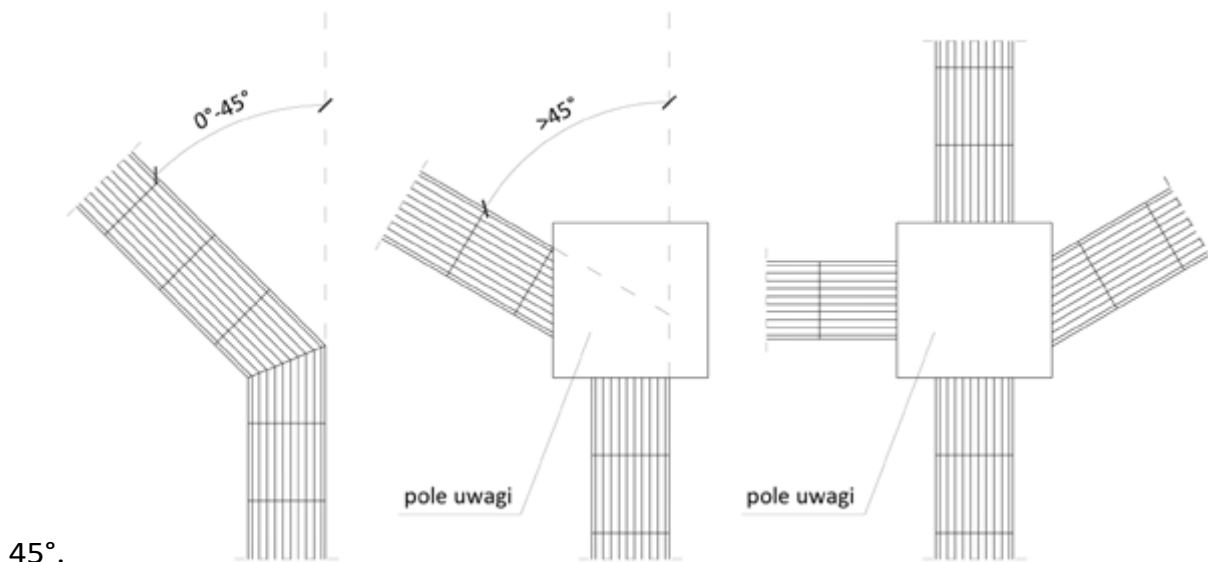
Ilustracja 11. Schemat łączenia ścieżek kierunkowych w miejscach zmiany kierunku ich przebiegu (po lewej i środku) oraz na skrzyżowaniach (po prawej), rys. Katarzyna Guratowska
