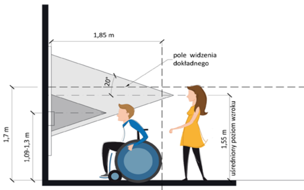
Ilustracja 95. Warunki dobrego widzenia dla użytkowników o zróżnicowanych potrzebach, rys. Agnieszka Sowińska i Maria Görlich-Opyd
