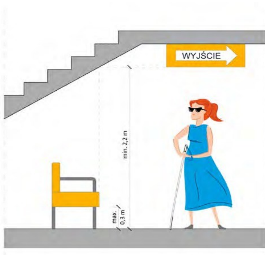
Ilustracja 64. Przykład zabezpieczenia przestrzeni pod schodami, rys. Katarzyna Guratowska i Maria Görlich-Opyd (opracowanie własne na podstawie „Modelu Dostępnej Szkoły”)
