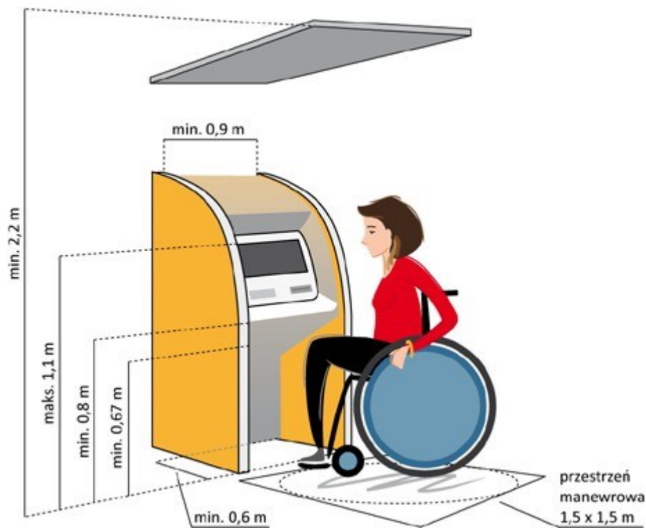
Ilustracja 34. Przykład kształtowania dostępnego automatu, rys. Maria Görlich-Opyd
