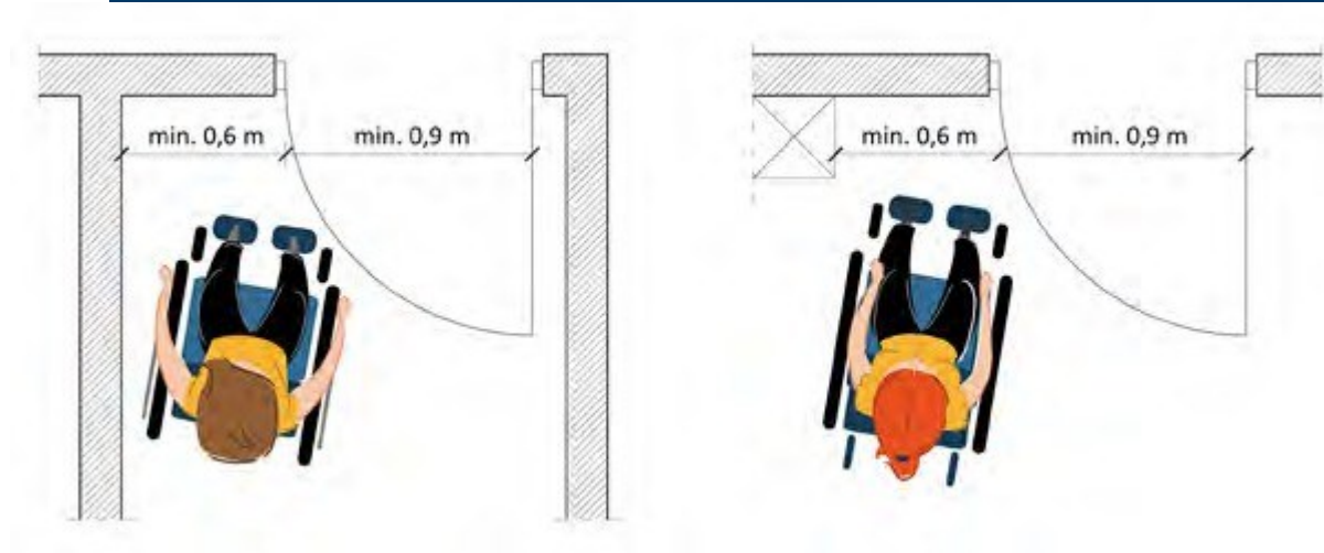
Ilustracja 62. Zasady zapewniania dostępu do drzwi w sposób umożliwiający ich samodzielne otwarcie, rys. Katarzyna Guratowska i Maria Görlich-Opyd (opracowanie własne na podstawie „Modelu Dostępnej Szkoły”)
