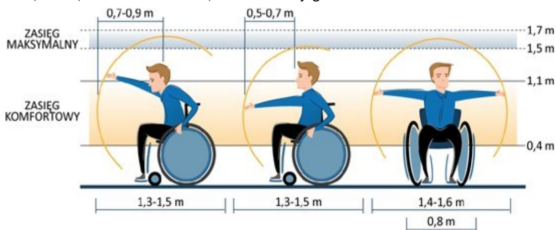
Ilustracja 3. Orientacyjny zasięg rąk użytkownika wózka, rys. Maria Görlich-Opyd
