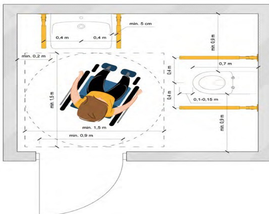
Ilustracja 77. Przykład rozmieszczenia sprzętów oraz powierzchni manewrowej i transferowej w toalecie przeznaczonej dla osób ze szczególnymi potrzebami, rys. Katarzyna Guratowska i Maria Görlich-Opyd (opracowanie własne na podstawie „Modelu Dostępnej Szkoły”)
