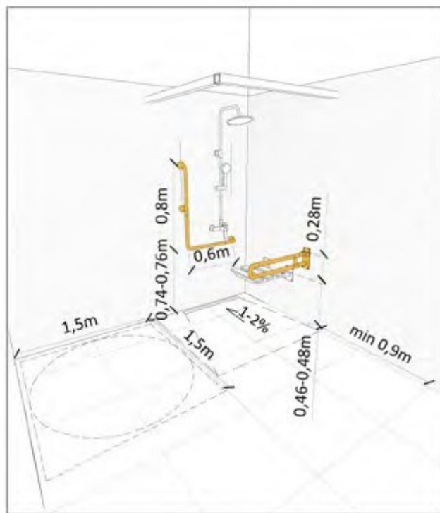
Ilustracja 80. Zasady montażu elementów wyposażenia prysznic w pomieszczeniach sanitarnych przeznaczonych dla osób ze szczególnymi potrzebami, rys. Agnieszka Sowińska (opracowanie własne na podstawie „Modelu Dostępnej Szkoły”)
