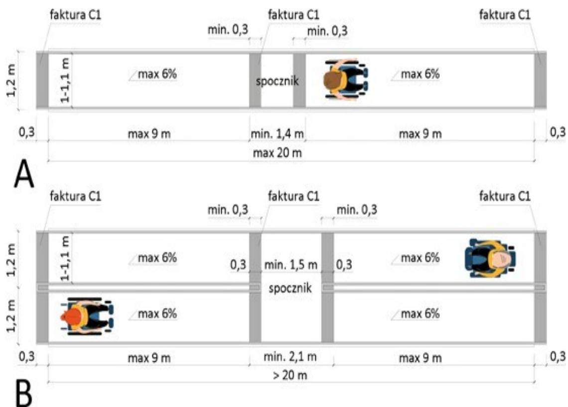
Ilustracja 49. Przykłady kształtowania pochylni zewnętrznych, A – pochylnia dwubiegowa z jednym pasem ruchu, B – pochylnia dwubiegowa z dwoma pasami ruchu, rys. Katarzyna Guratowska i Maria Görlich-Opyd
