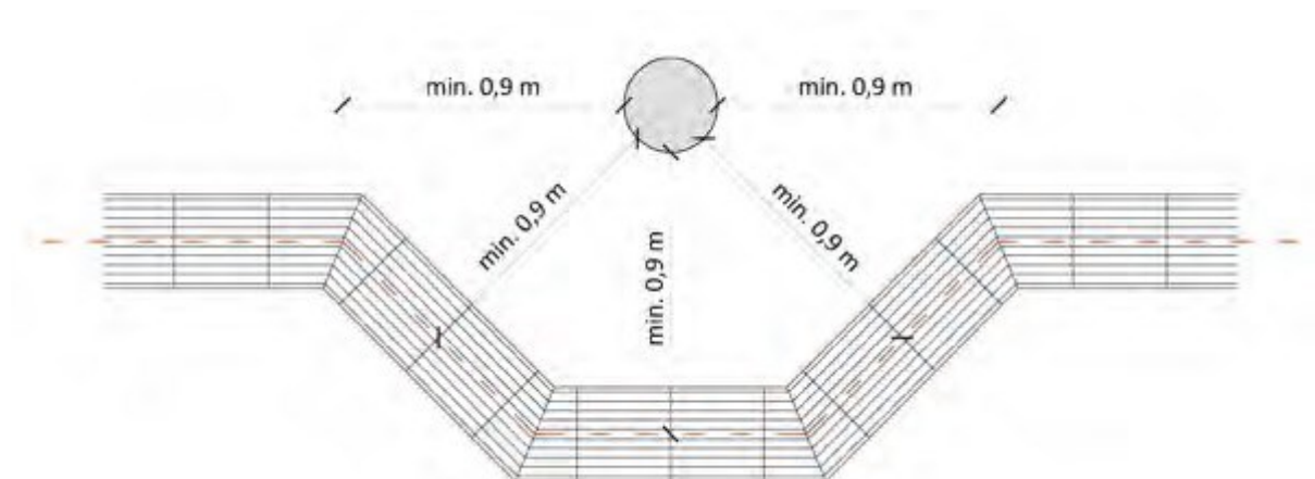
Ilustracja 13. Schemat prowadzenia ścieżek kierunkowych w pobliżu przeszkód, rys. Katarzyna Guratowska
