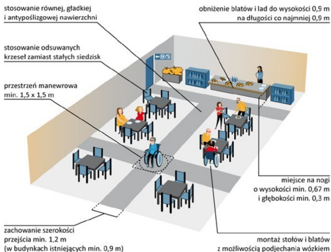
Ilustracja 92. Przykład aranżacji stołówki lub sali restauracyjnej, rys. Maria Görlich-Opyd
