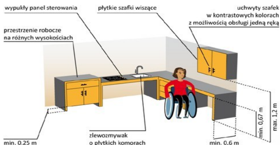
Ilustracja 91. Przykład aranżacji aneksu kuchennego, rys. Maria Görlich-Opyd Wyposażenie stołówki lub miejsc służących spożywaniu posiłków
