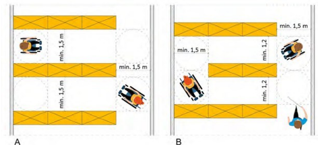
Ilustracja 88. Przykłady kształtowania przejść między regałami w bibliotece lub archiwum, rys. Katarzyna Guratowska i Maria Görlich-Opyd (opracowanie własne na podstawie „Modelu Dostępnej Szkoły”)
