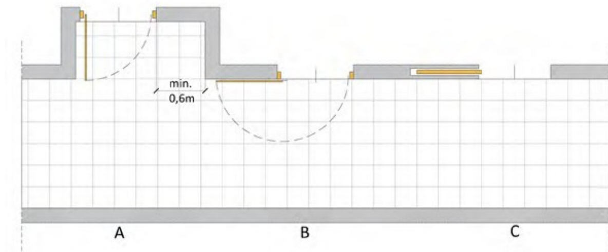
Ilustracja 59. Zasady sytuowania drzwi w przestrzeni korytarza w sposób niezagrażający użytkownikom: A – drzwi rozwierane pod kątem 90° sytuowane w wnękach, B – drzwi rozwierane pod kątem 180°, C – drzwi rozsuwane, rys. Agnieszka Sowińska (opracowanie własne na podstawie „Modelu Dostępnej Szkoły”).
