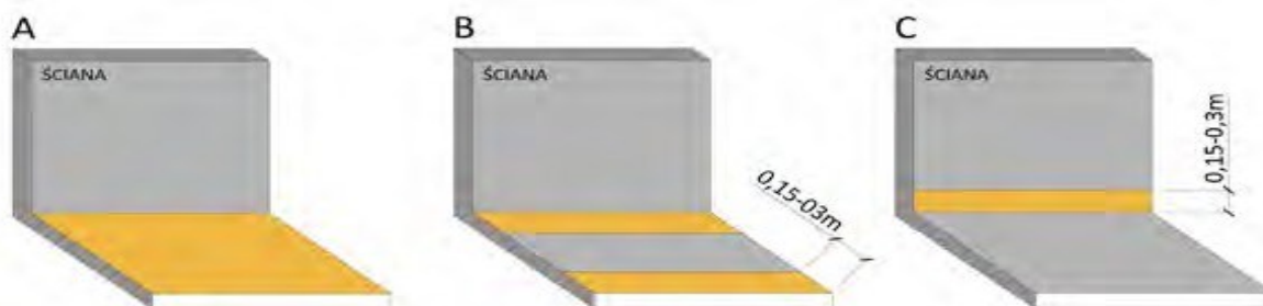
Ilustracja 57. Sposób kontrastowania kolorystycznego ściany i posadzki: A – zróżnicowanie barw obu płaszczyzn, B – wprowadzenie na posadzce pasa w kontrastowym kolorze, C – wprowadzenie cokołu na ścianie w kontrastowym kolorze, Agnieszka Sowińska (opracowanie własne na podstawie „Modelu Dostępnej Szkoły”)
