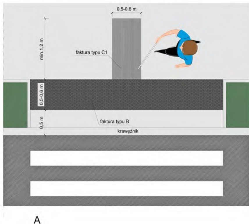
Ilustracja 25. Zasady stosowania pasów ostrzegawczych przy przejściach dla pieszych – przykład pasa ostrzegawczego odsuniętego od krawędzi jezdni, rys. Katarzyna Guratowska i Maria Görlich-Opyd
