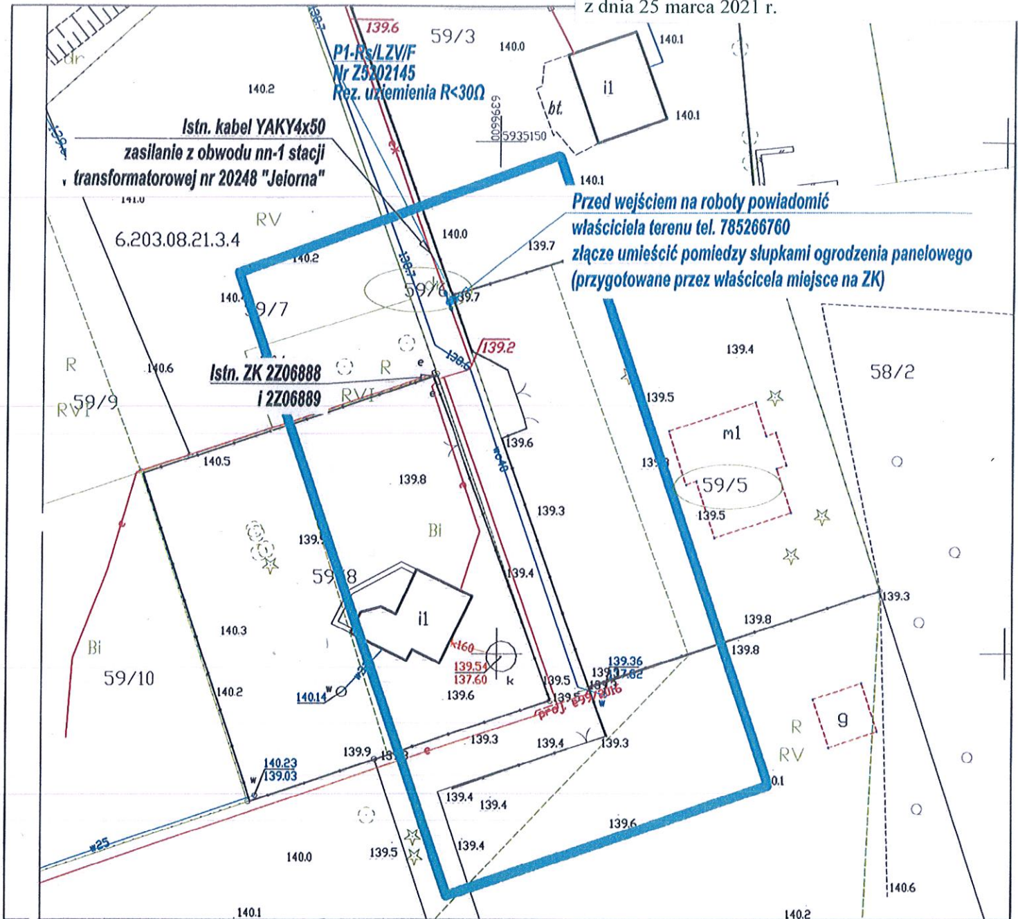
SZCZEGÓL SKALA 1:200
