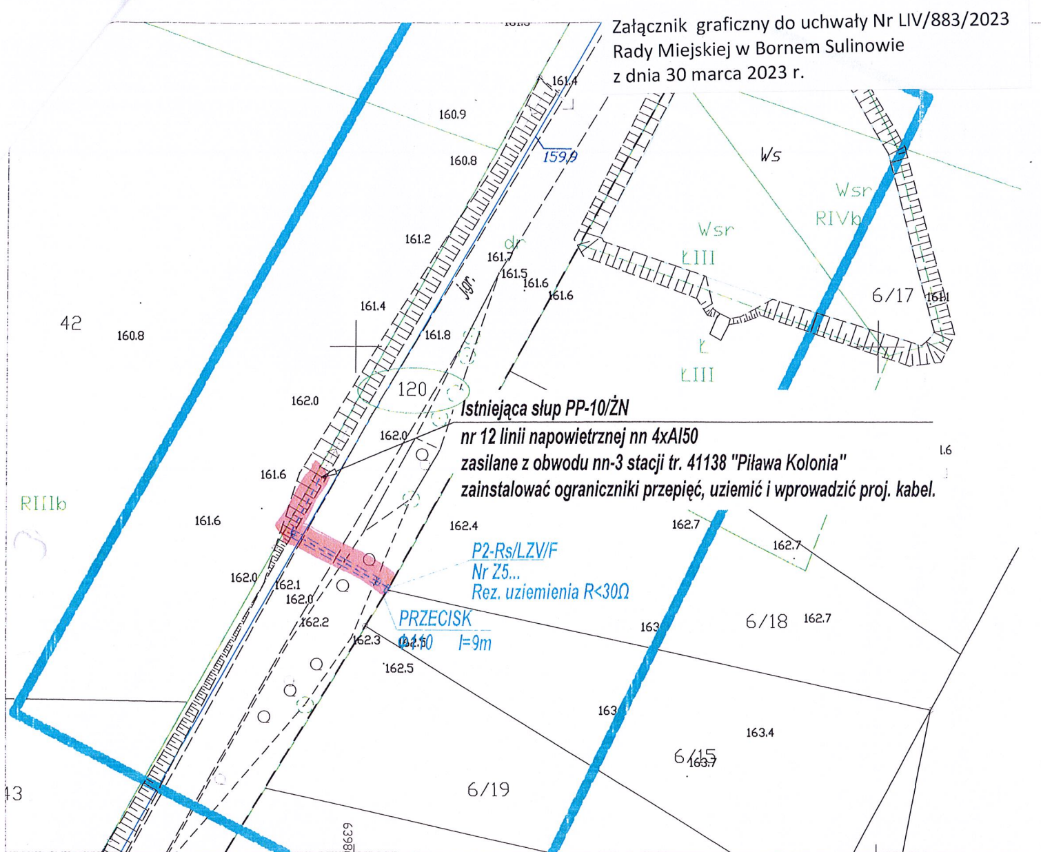
Szczegół, SKALA 1:200
