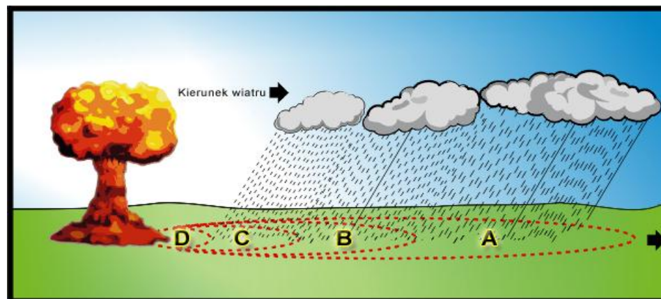
Rozprzestrzenianie się fali uderzeniowej i pyłu radioaktywnego podczas wybuchu jądrowego.
